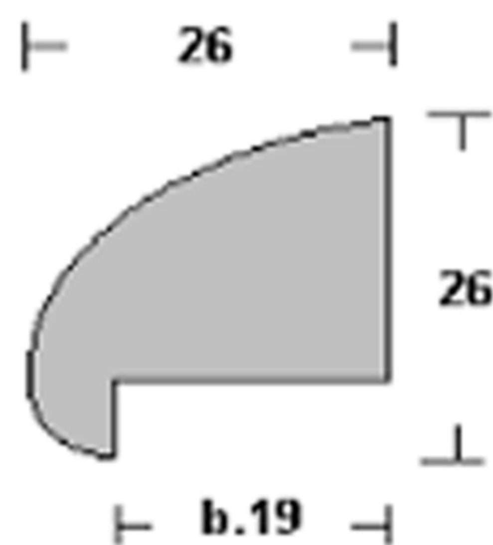
Art. 36 - 1T 26 x 26
